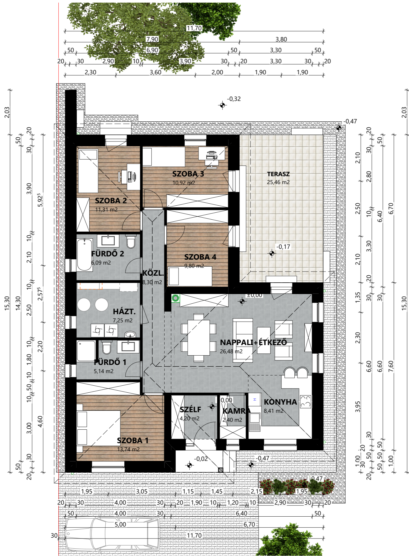
L5 Ház Nettó alapterület: 114 m 2 + Terasz
