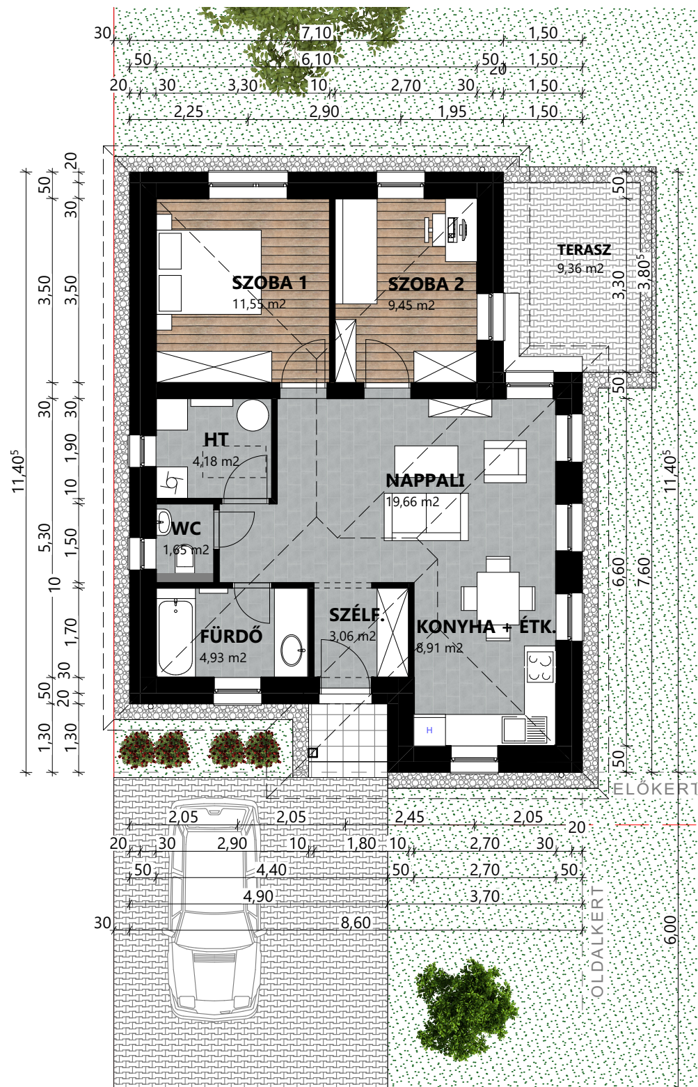
L11 Ház Nettó alapterület: 63,39 m 2 + Terasz
